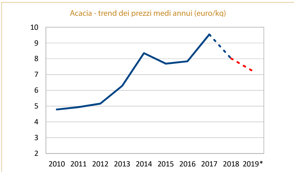
Grafico 1. Andamento dei prezzi medi annui del miele di acacia convenzionale. La linea continua blu esprime l'andamento dei prezzi medi annui registrati dal 2010 al 2019. La linea tratteggiata blu esprime la tendenza negativa registrata per il 2018 e la linea tratteggiata rossa esprime l'ulteriore trend negativo stimato dal 2018 al 2019.
