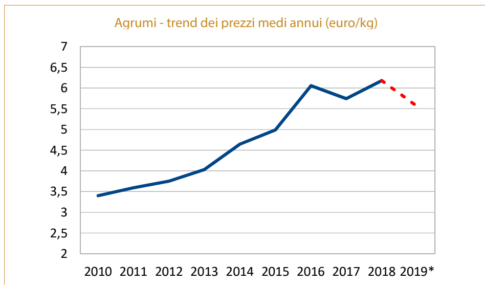
Grafico 2. Andamento dei prezzi medi annui del miele di agrumi convenzionale. La linea continua blu esprime l'andamento dei prezzi medi annui registrati dal 2010 al 2019. La linea tratteggiata rossa esprime il trend negativo stimato dal 2018 al 2019.
