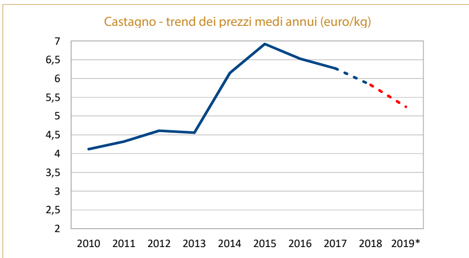
Grafico 3. Andamento dei prezzi medi annui del miele di castagno convenzionale. La linea continua blu esprime l'andamento dei prezzi medi annui registrati dal 2010 al 2019. La linea tratteggiata blu esprime la tendenza negativa registrata per il 2018 e la linea tratteggiata rossa esprime l'ulteriore trend negativo stimato dal 2018 al 2019.
